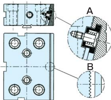
プリズムコーム口金の寸法
